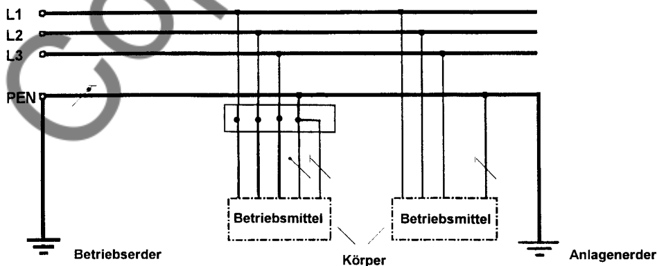
Bild 3-2: TN-C-System (PE-Leiter und Neutraleiter im gesamten System als PEN-Leiter zusammengefasst)
